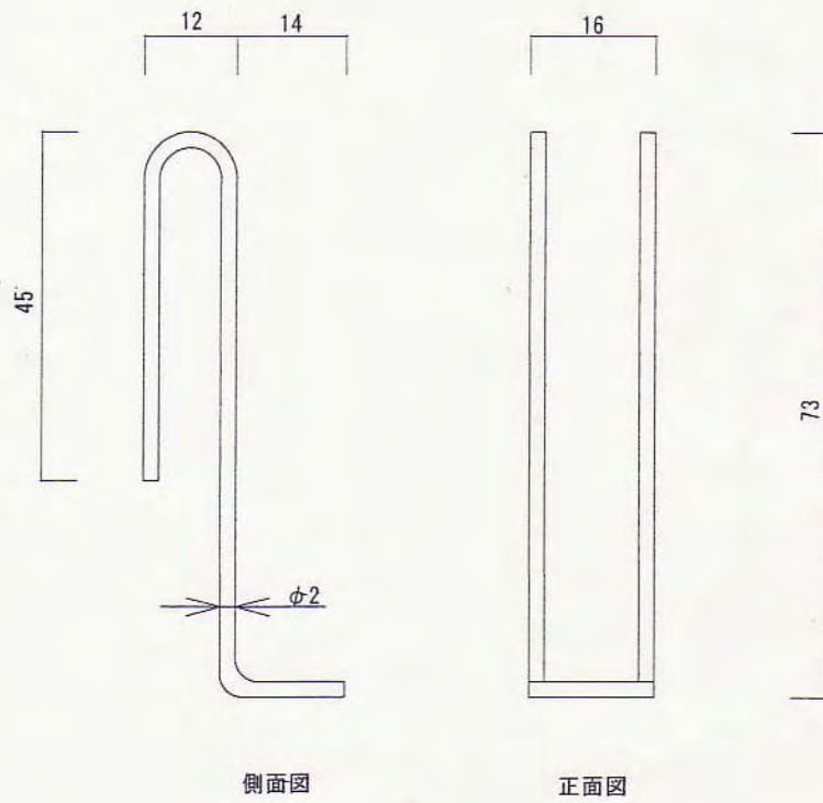
受け金具
