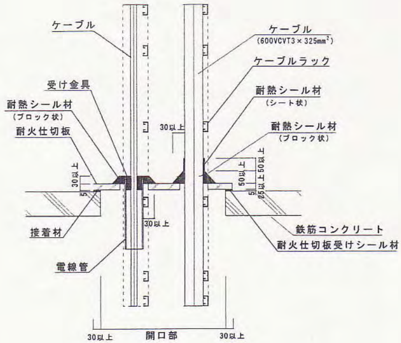
A-A' 断面図
